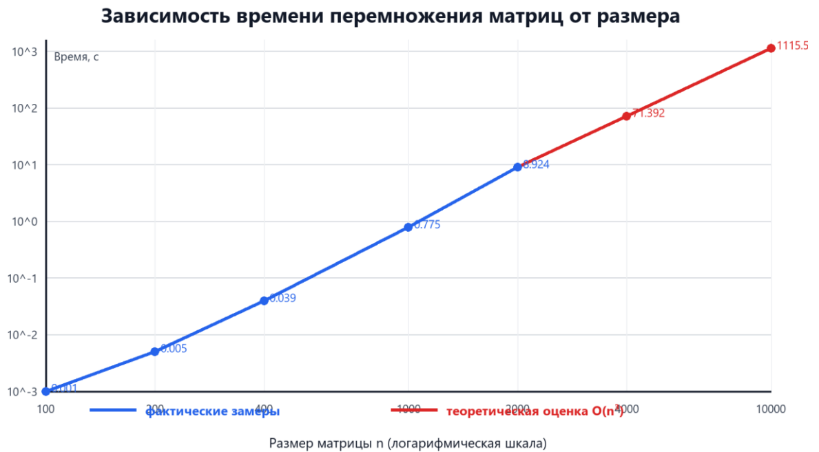
Рисунок 1 — График зависимости времени перемножения матриц от размера
